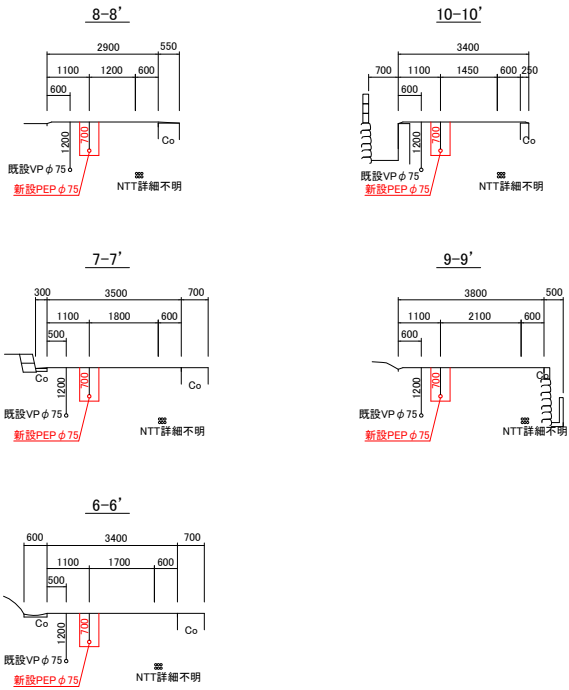
横断面図1 S=1/500
