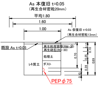
消火栓土工図
