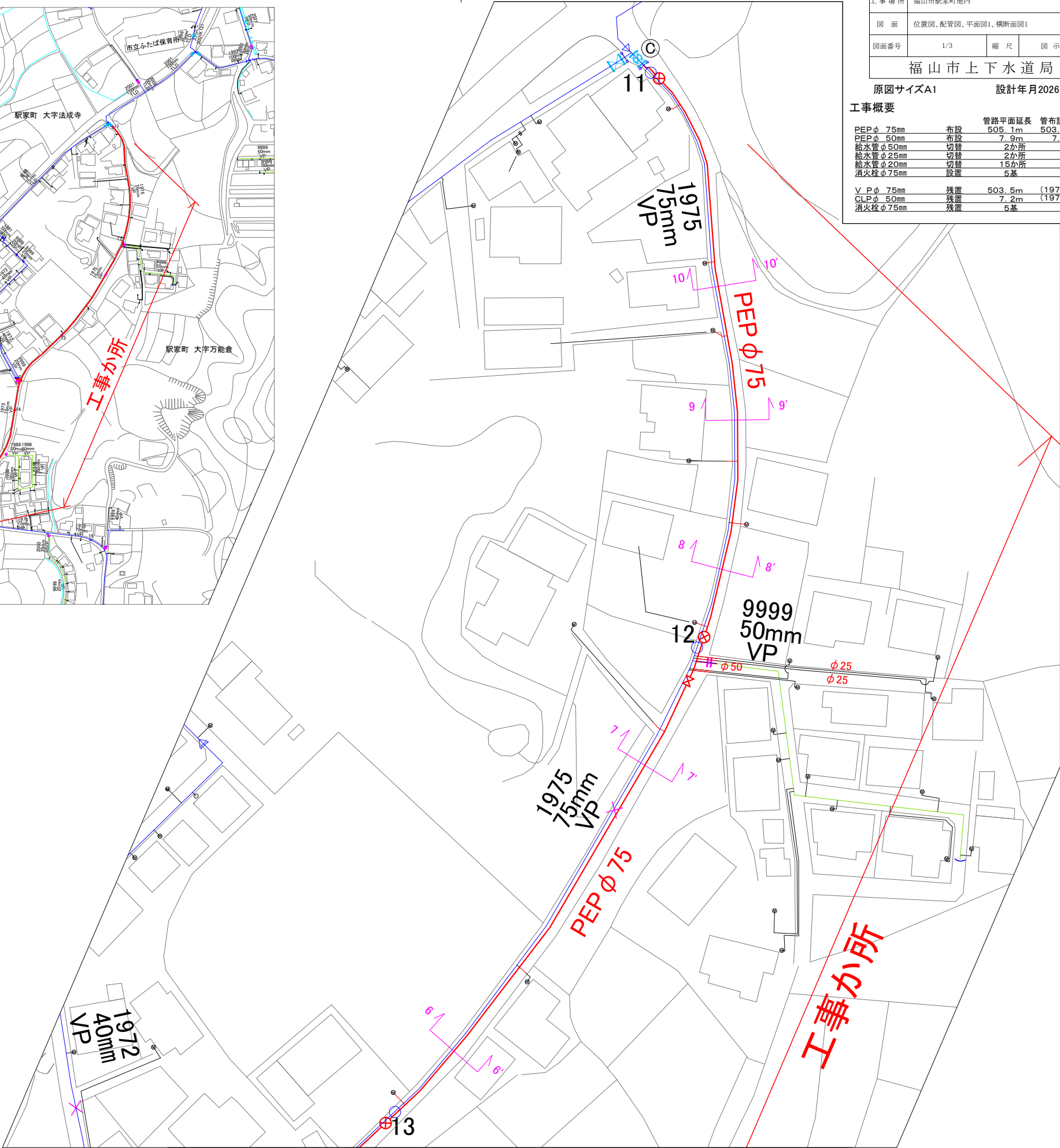
平面図1 S=1/500
