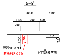
横断面図2 S=1/500
