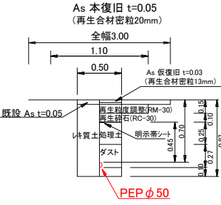
PEP φ 50土工図
