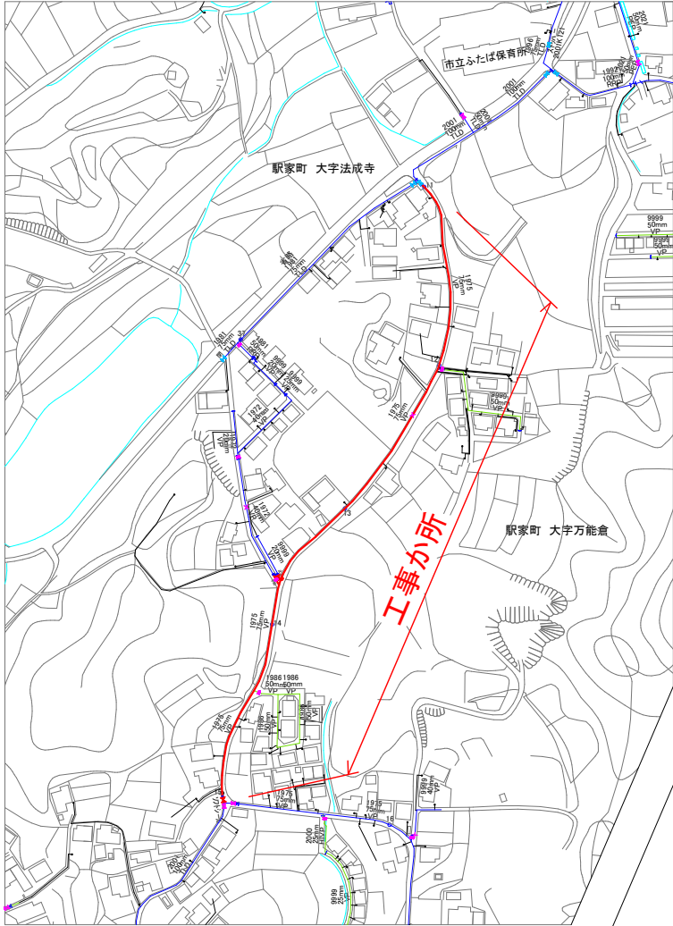
配管図 S=1/2500
