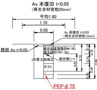
PEP φ 75土工図
