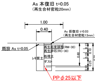
給水管 φ 25以下土工図
