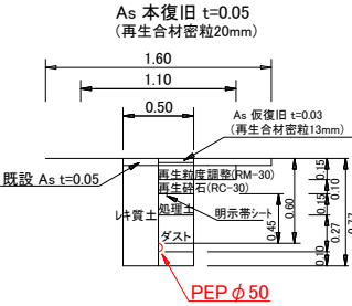
給水管 φ 50土工図
