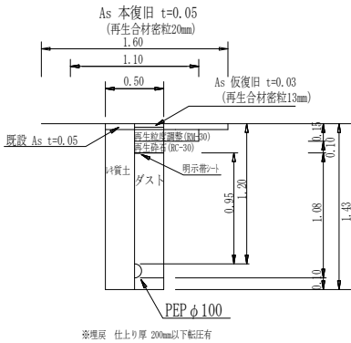
PEP φ100土工図
