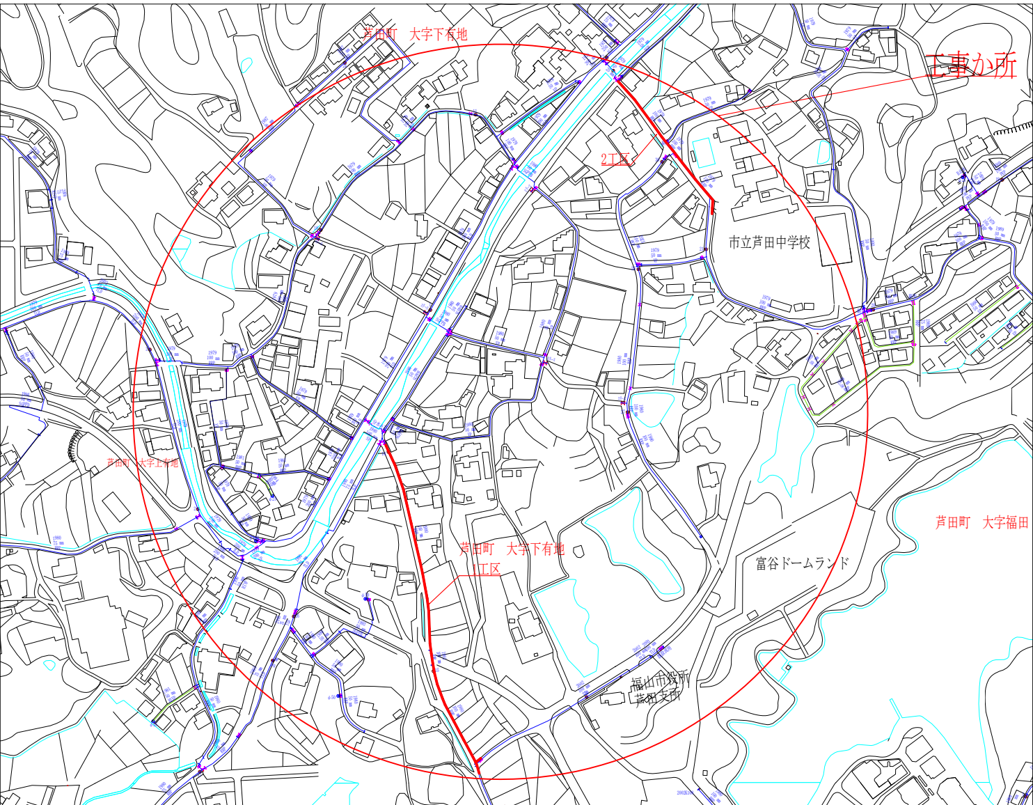
配管図 S=1/2,500
