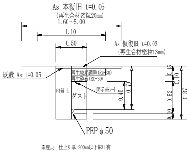
ドレン φ50土工図 PEP φ50土工図
