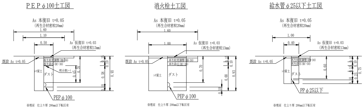
土工図 S=1/30
