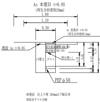
給水管 φ50土工図
