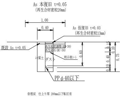
給水管 φ40以下土工図
