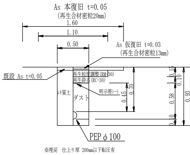
PEP φ100土工図
