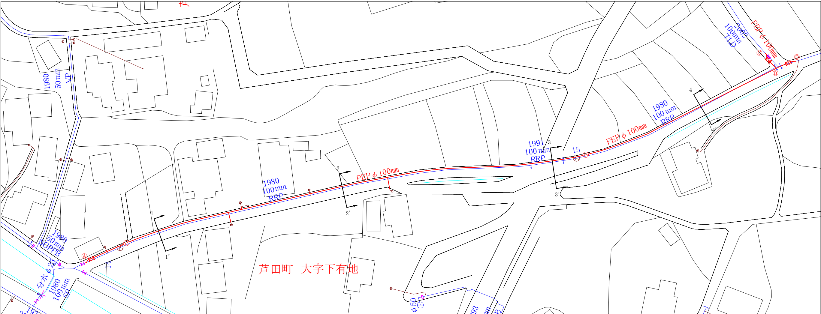
平面図【1工区】 S=1/500
