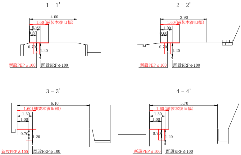
横断面図 S=1/100
