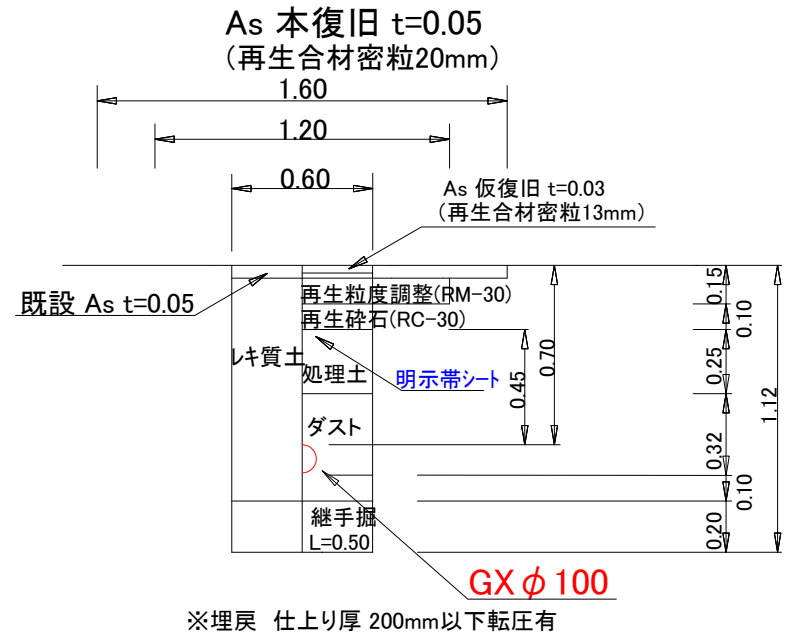
GXφ100土工図①
