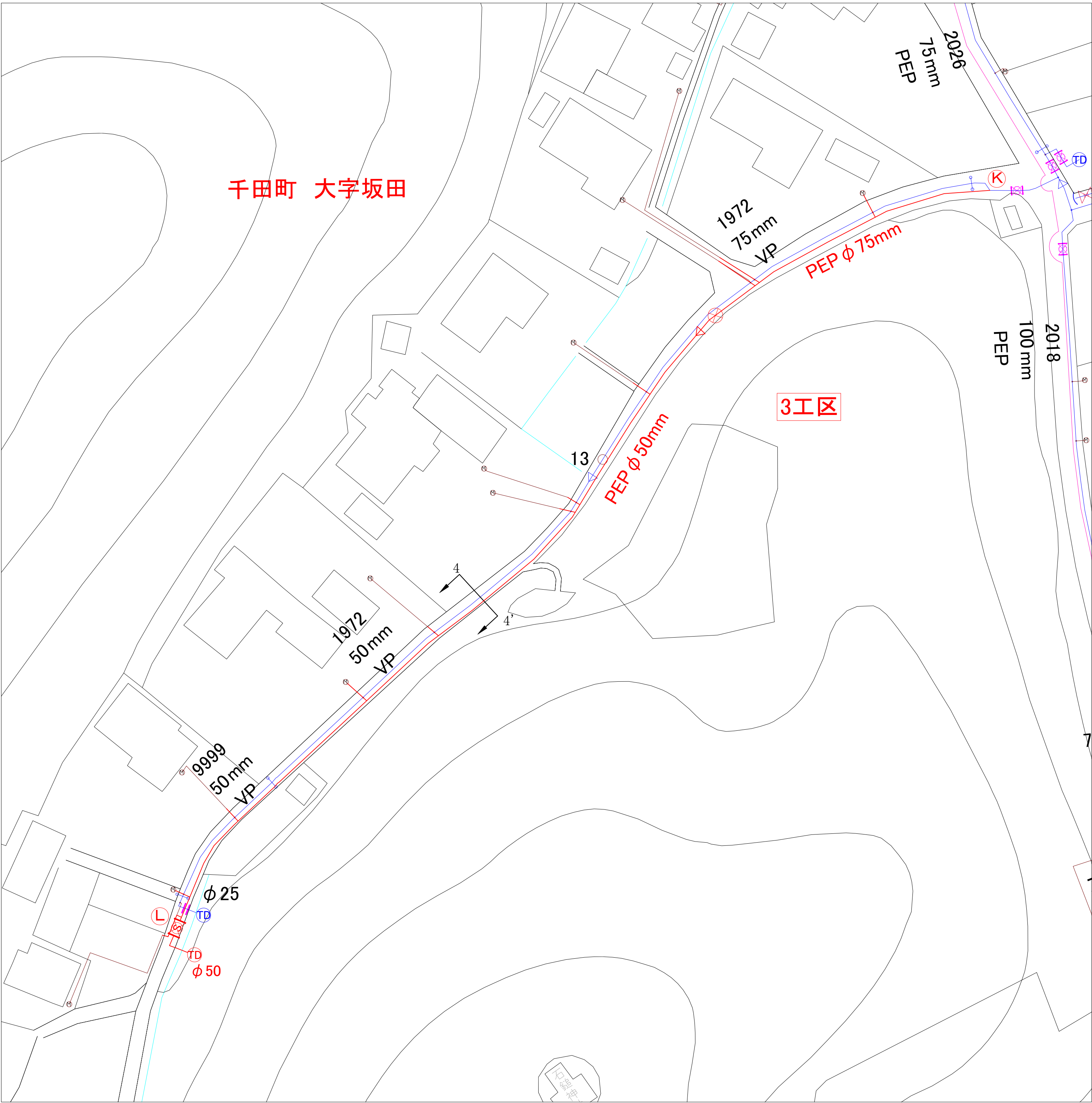
平面図(3工区) S=1/500
