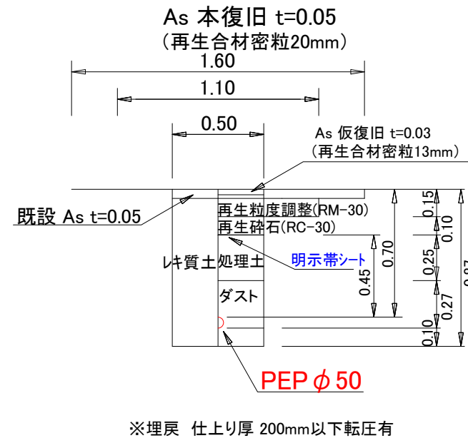
PEPφ50・ドレンφ50土工図④
