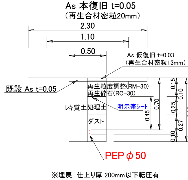
PEPφ50・ドレンφ50土工図⑤
