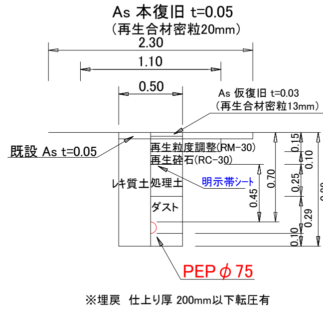
PEPφ75土工図③
