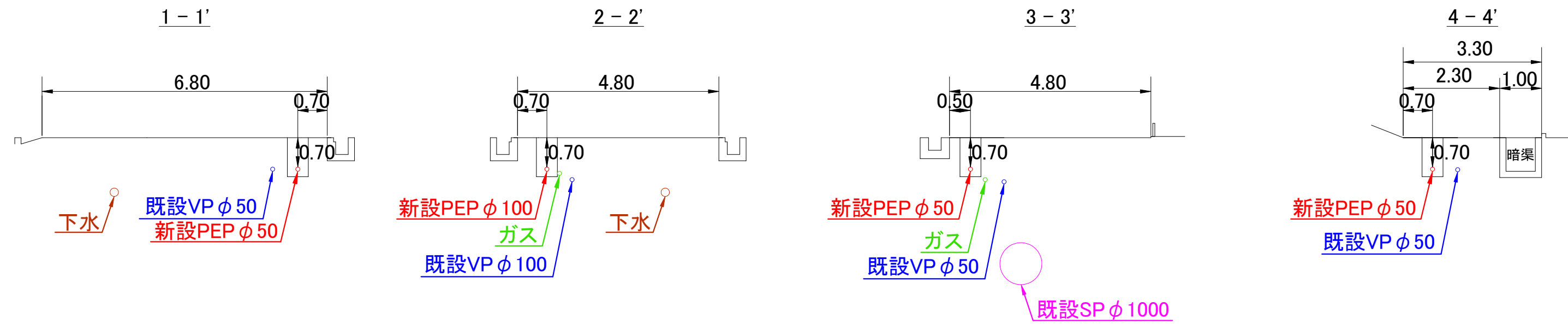
横断面図 S=1/100
