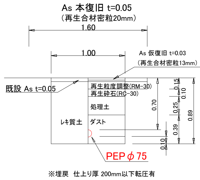
消火栓土工図⑥
