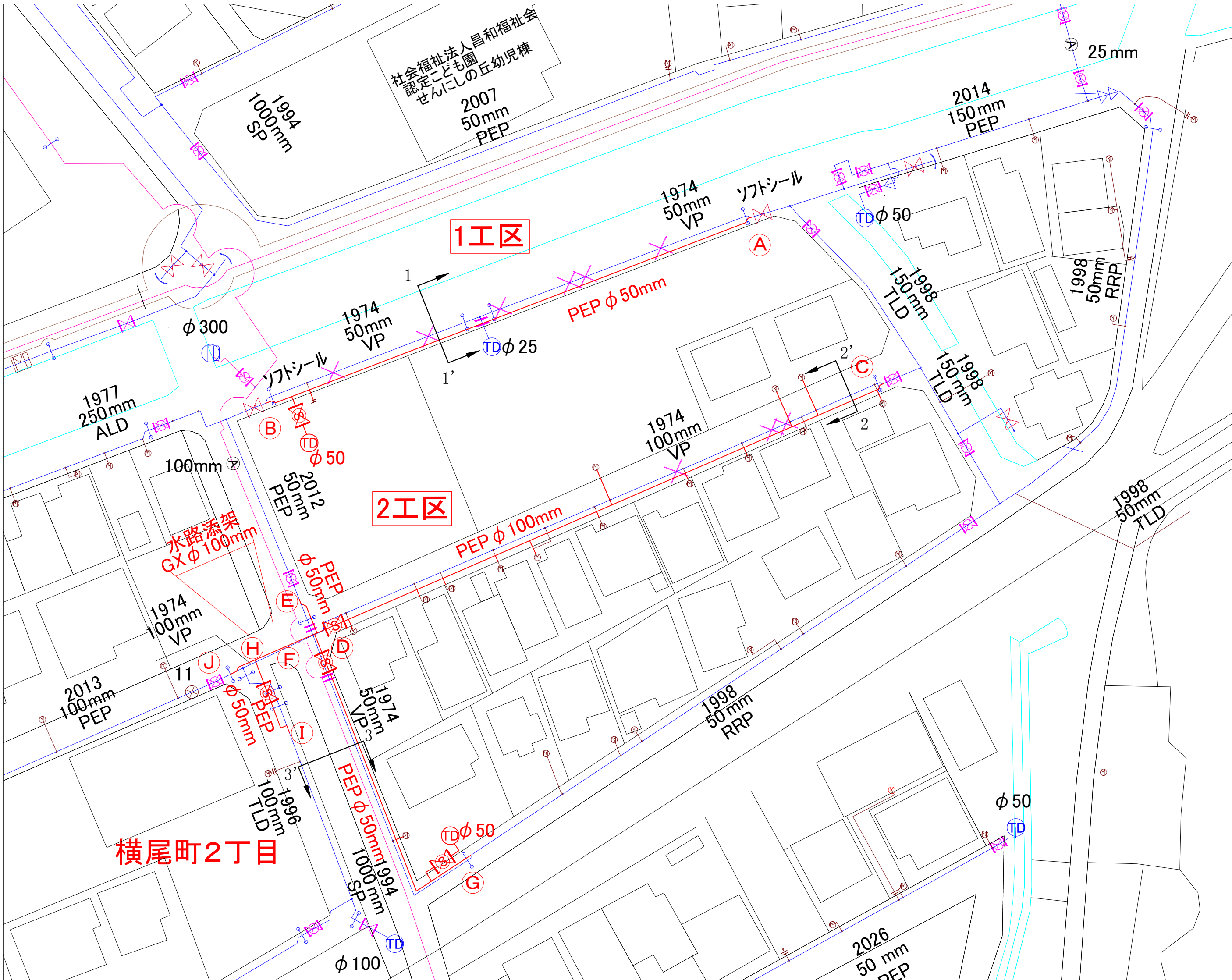
平面図(1~2工区) S=1/500
