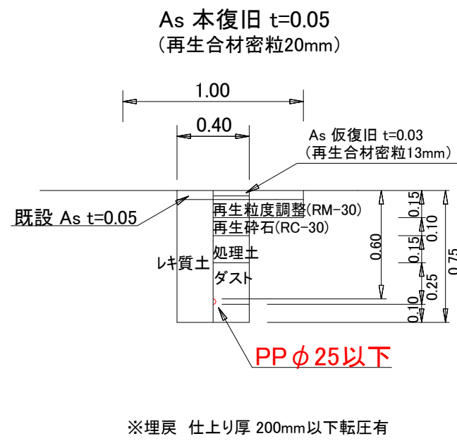
給水管φ25以下土工図⑦
