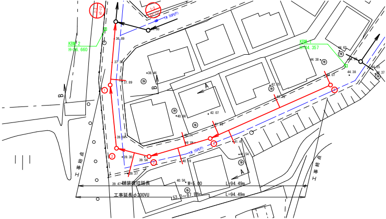
管渠埋設縦断面図
