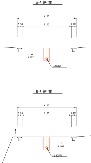
管渠埋設断面図
