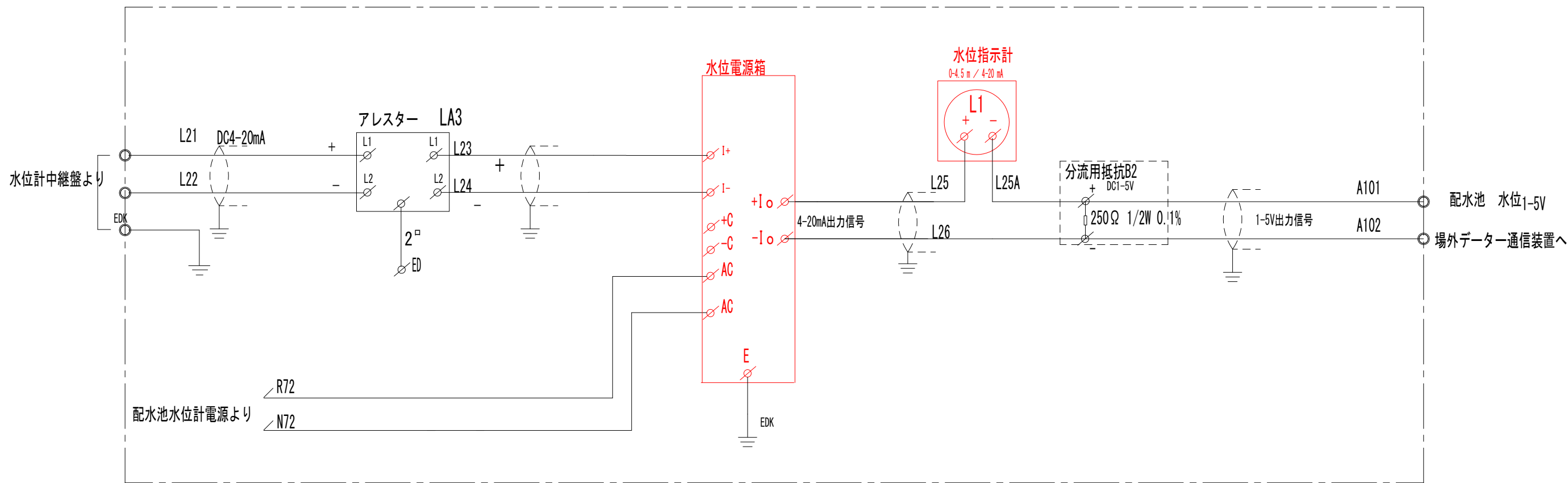
計装ループ図（改修後）
