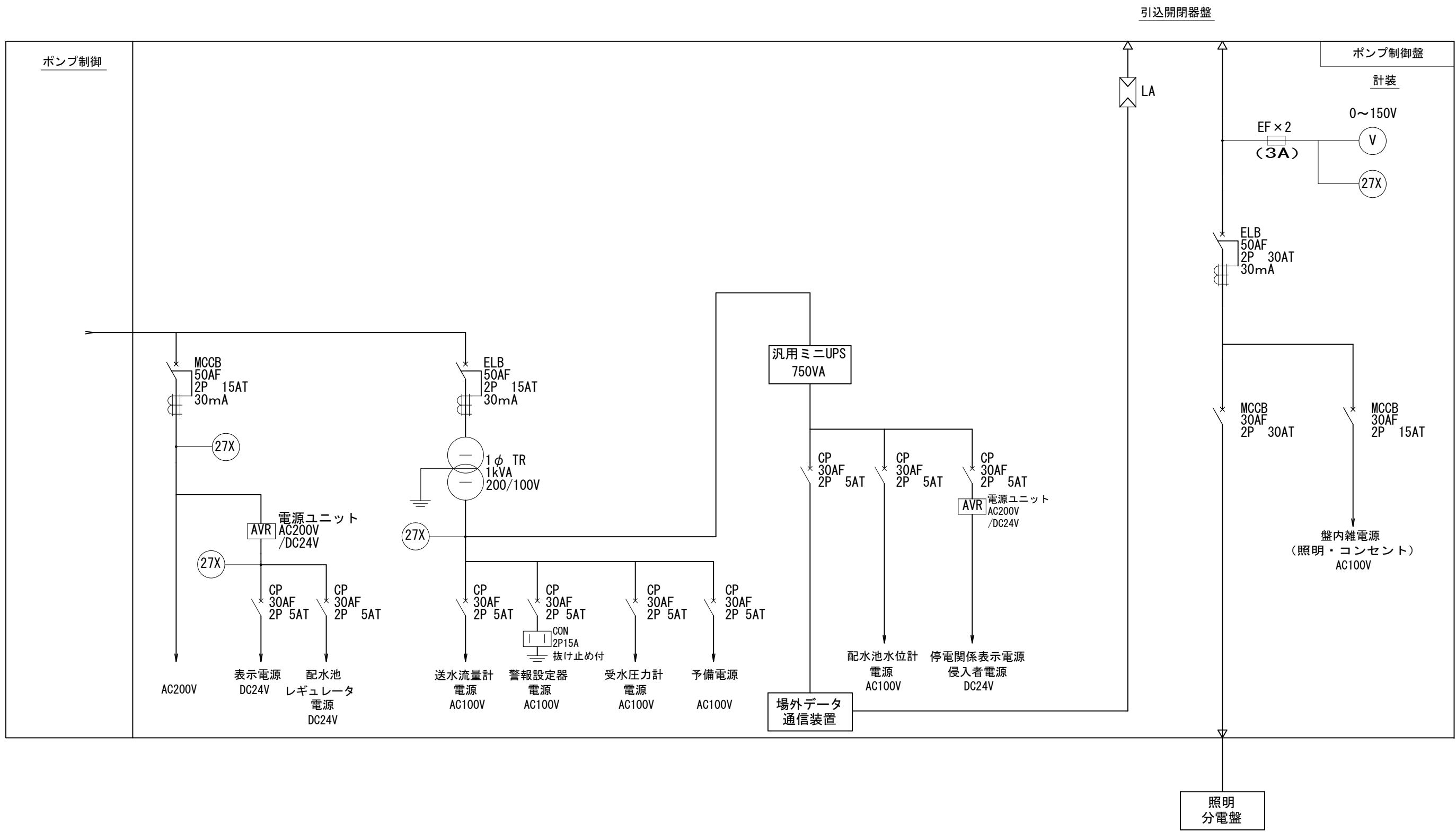
ポンプ制御盤単線結線図（改修前）
