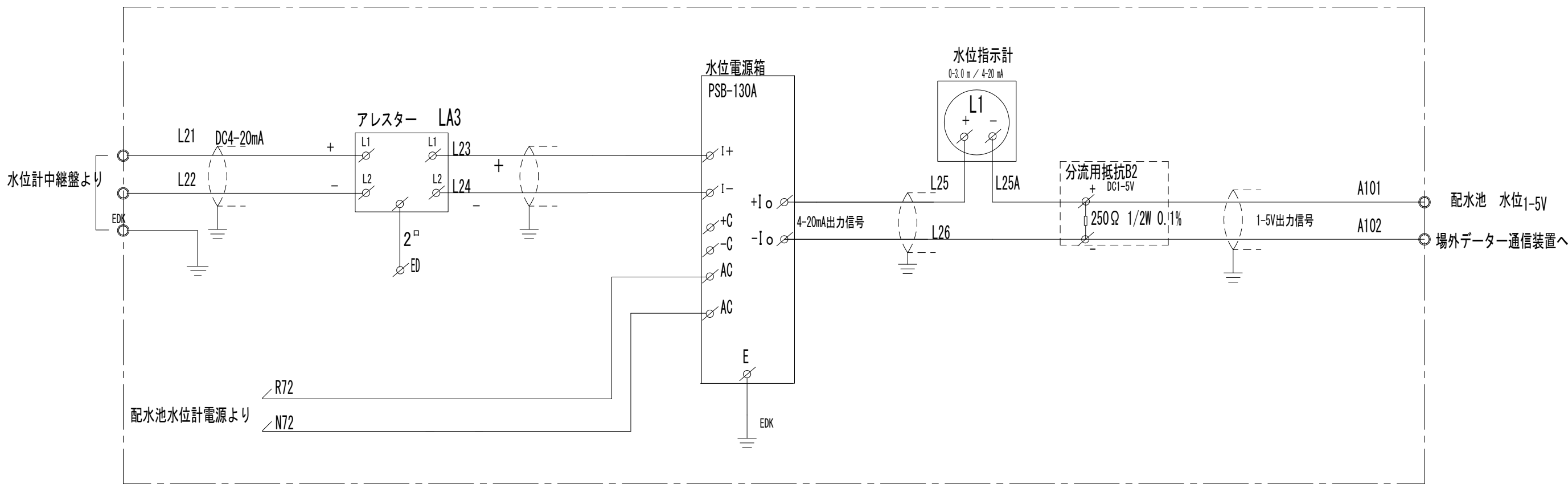
計装ループ図（改修前）
