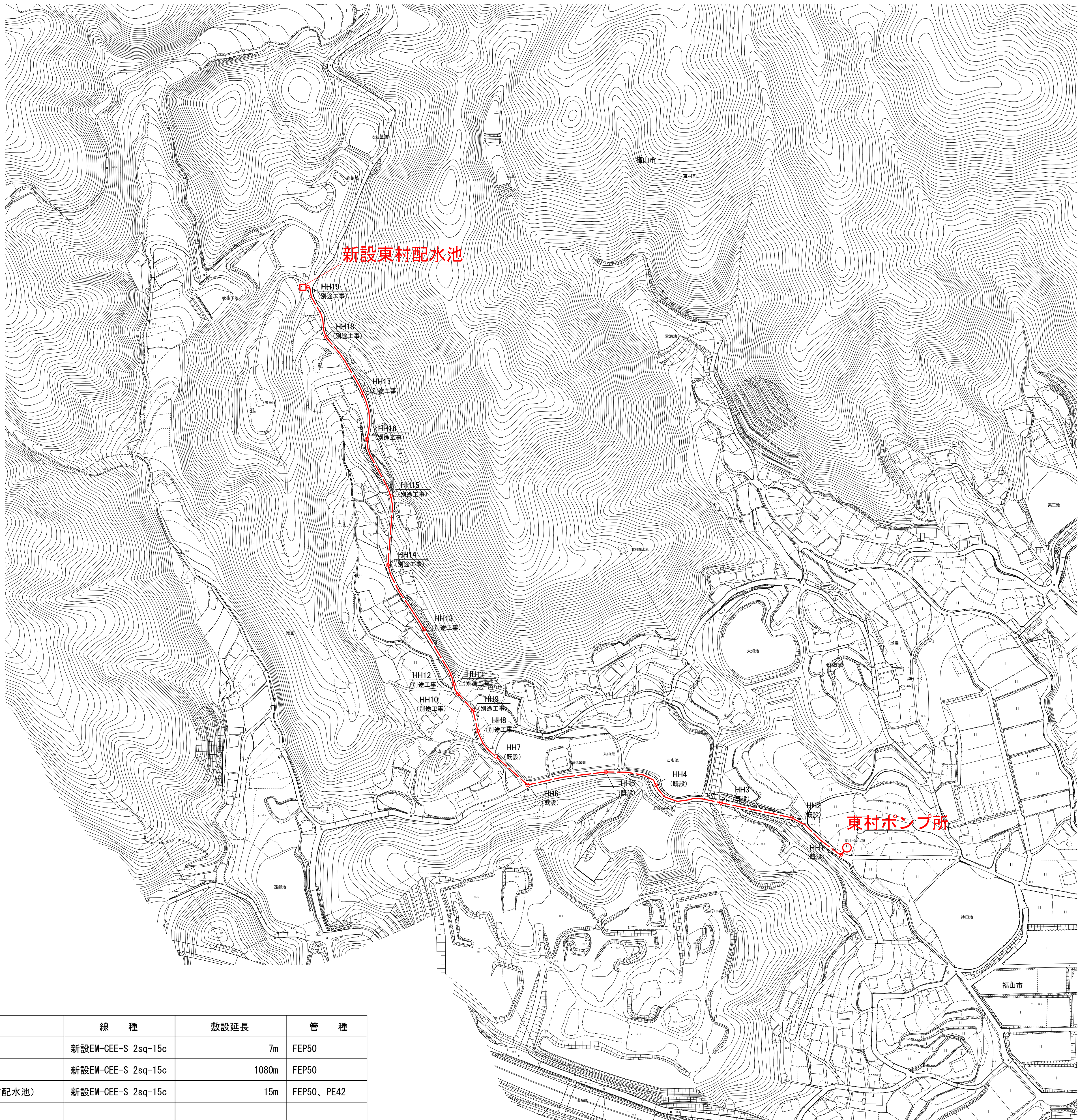
全体平面図 S=1/2,500
