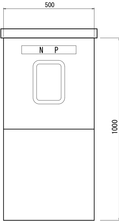
正面図 S=1/10
