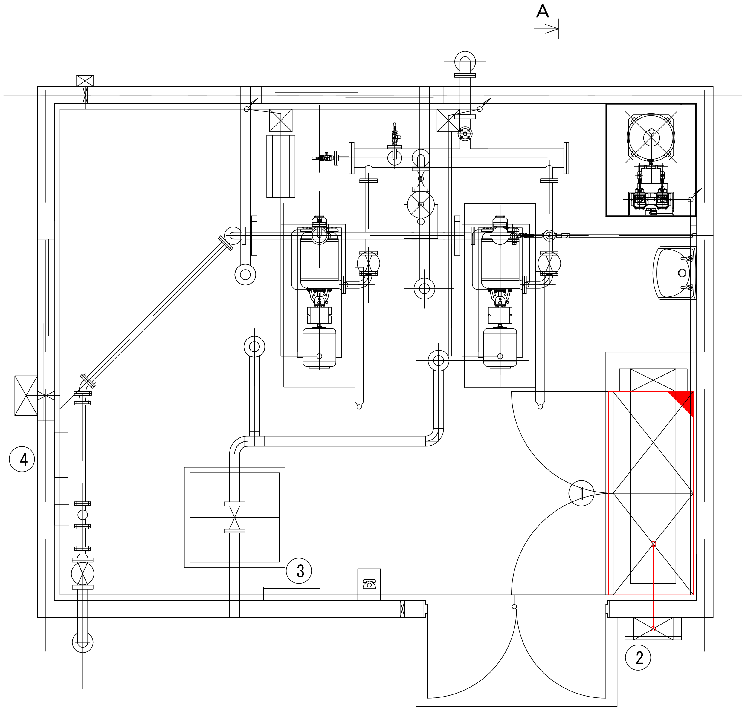
ポンプ室平面図
