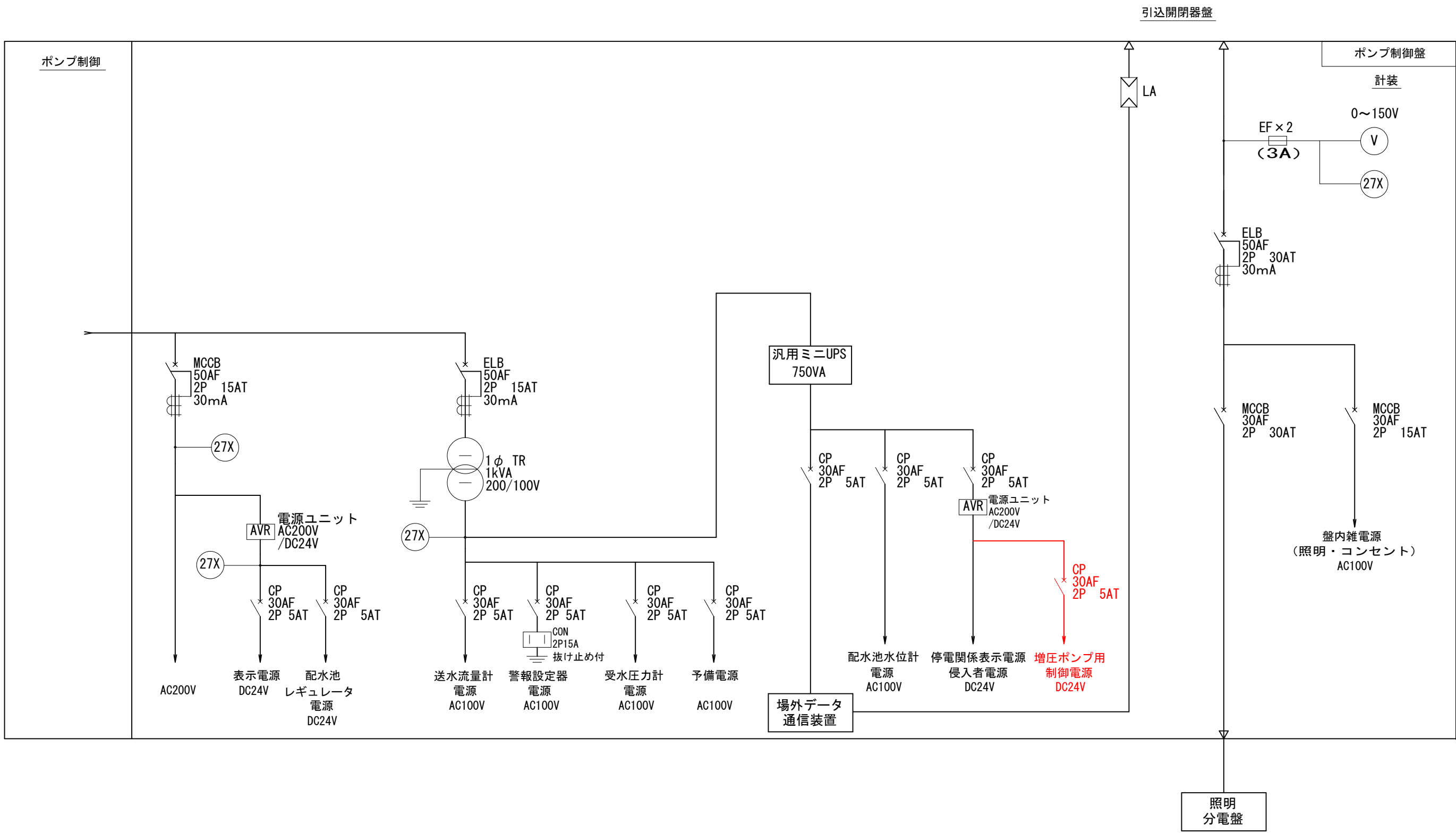
ポンプ制御盤単線結線図（改修後）
