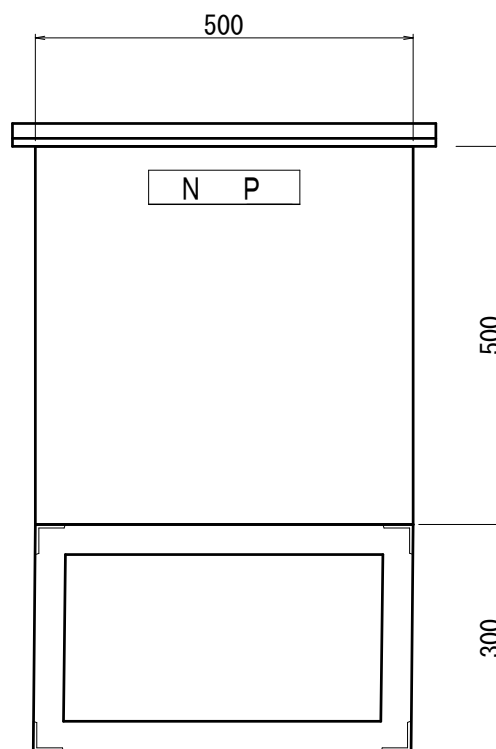
正面図 S=1/10
