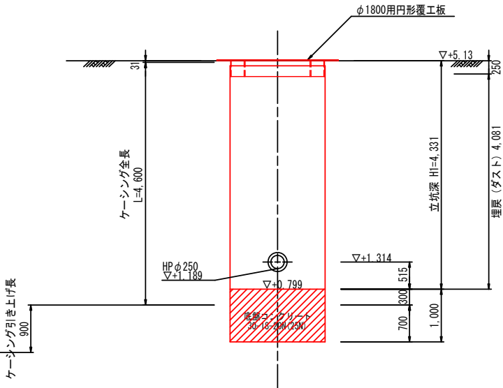
立坑構築完了図
