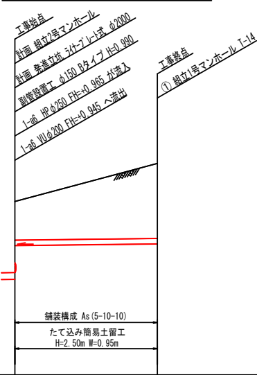
管渠埋設縦断面図 Y=1:100 H=1:500
