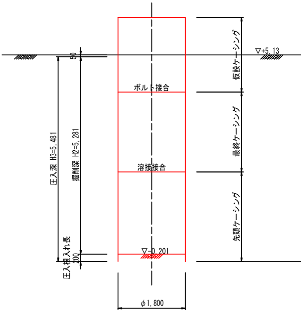
圧入掘削完了図
