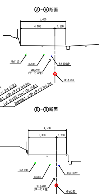
管渠埋設横断面図 S=1:100
