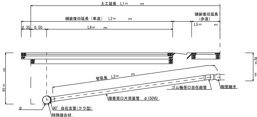
取付管埋設縦断面図
