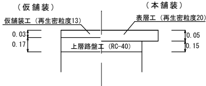
舗装復旧断面図 (歩道)
