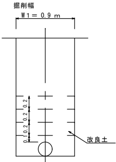
管埋設断面図
