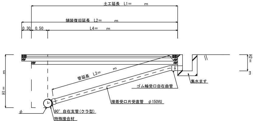
取付管埋設縦断面図
