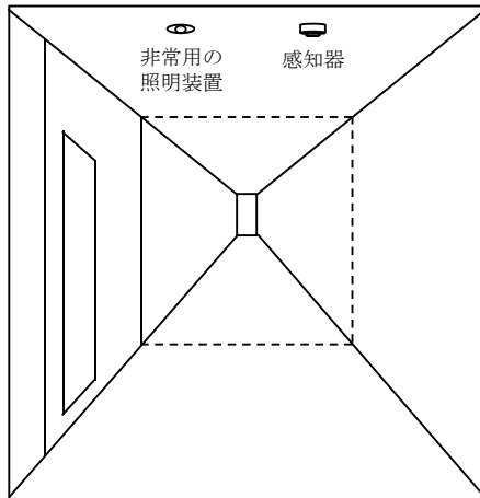
&lt;感知器連動閉鎖式防火戸（平常時）&gt;
