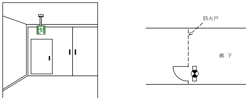
< 廊下等に防火戸がある場合の設置例 >
