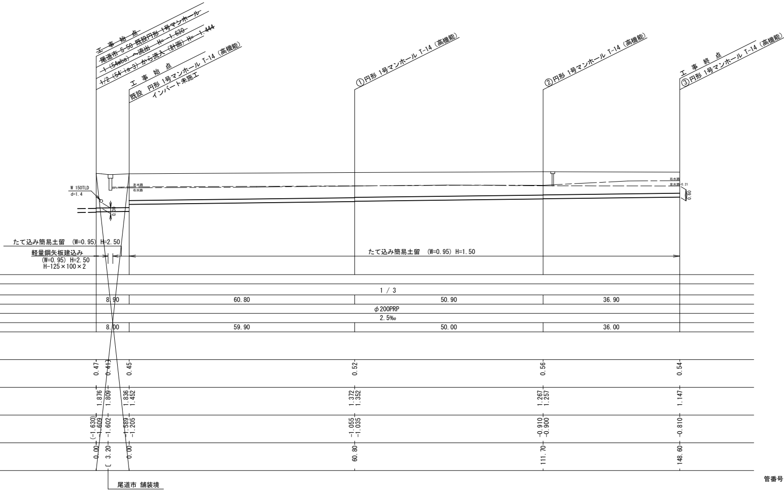
管渠埋設縦断面図 S = 縦横 1:100 1:500
