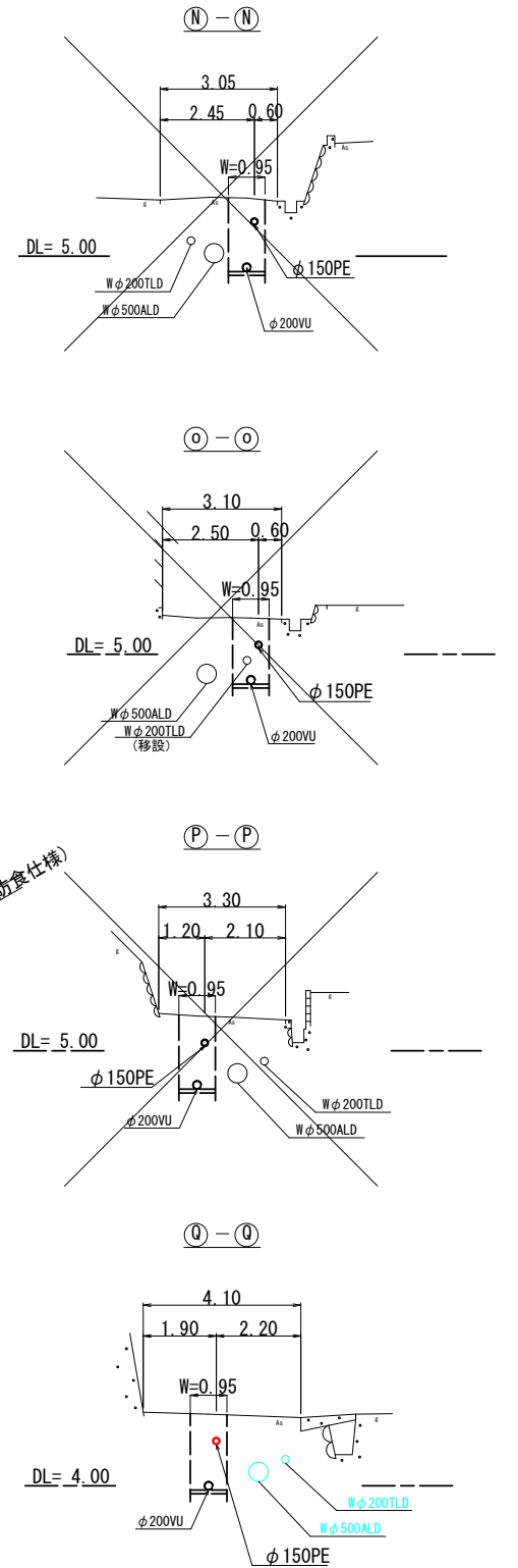
標準横断面図 S=1/100
