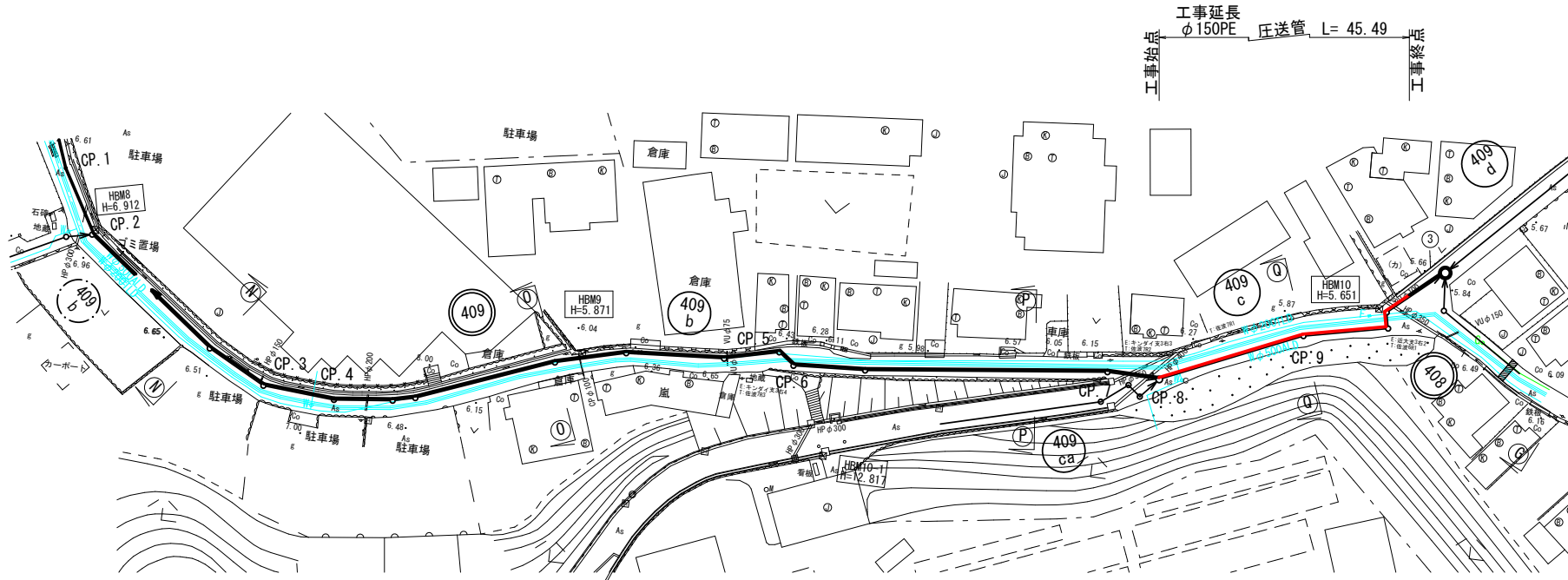
管渠埋設平面図 S=1/500
