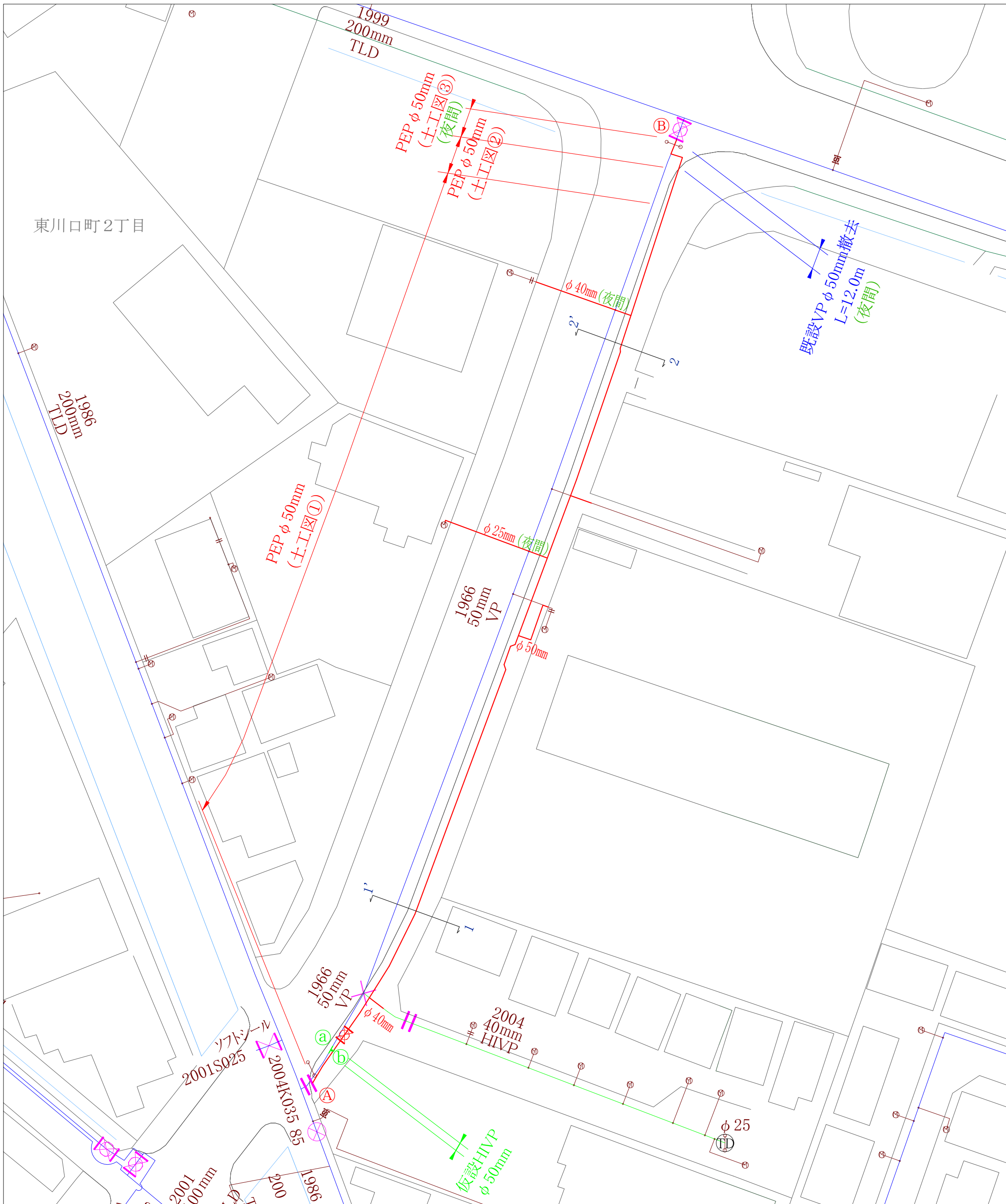
平面図 S=1/500
