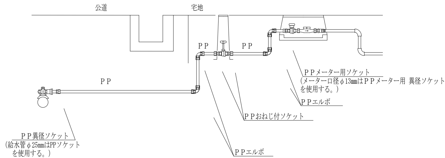
給水管切替標準施工図 S=NON
