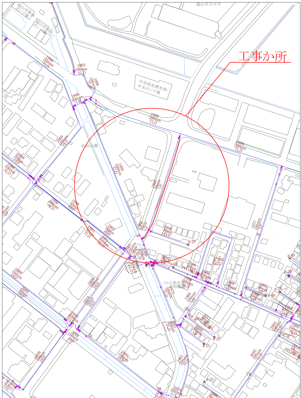
配管図 S=1/2500
