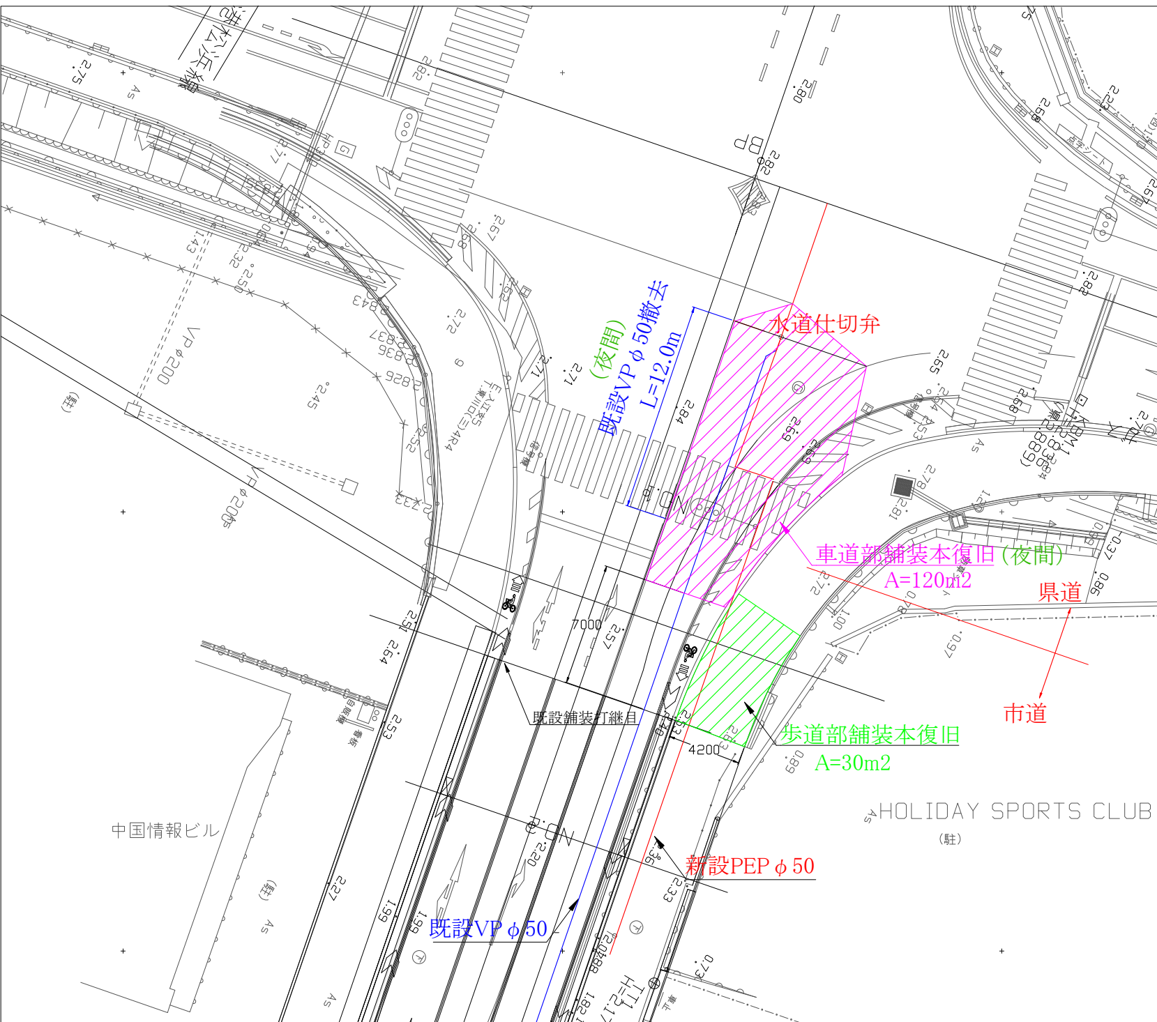
舗装本復旧平面図 S=1/300
