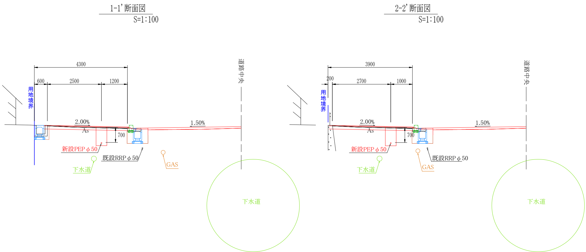
横断面図 S=1/100
