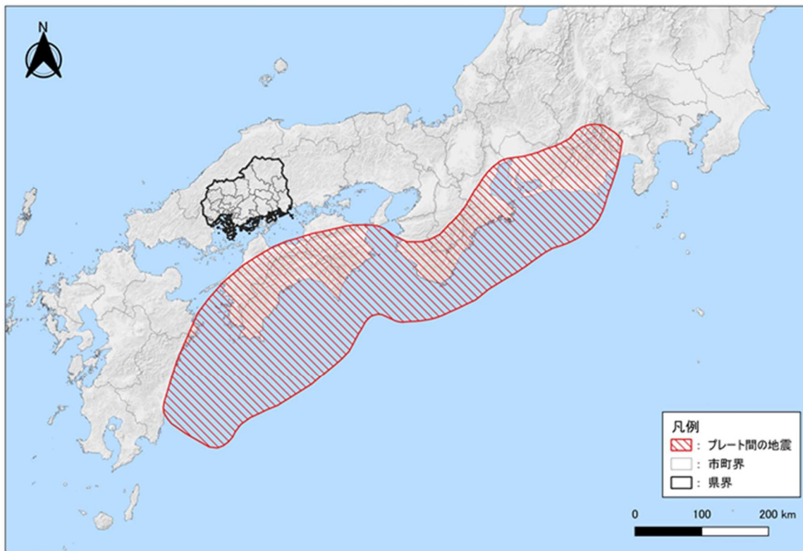
図ー1 想定地震位置図（南海トラフ巨大地震）
