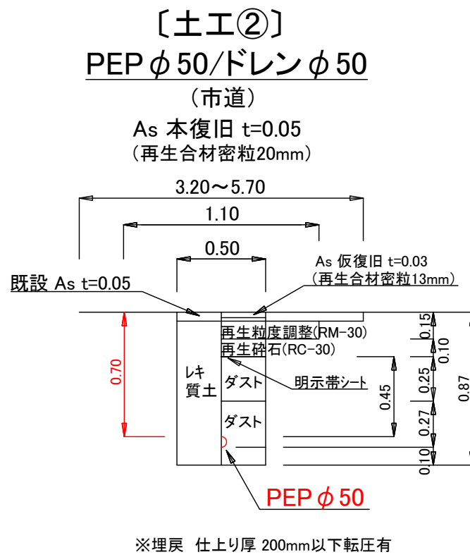
標準土工図 S=1/30
