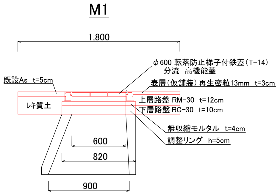
マンホール蓋取替詳細図 S=NON
