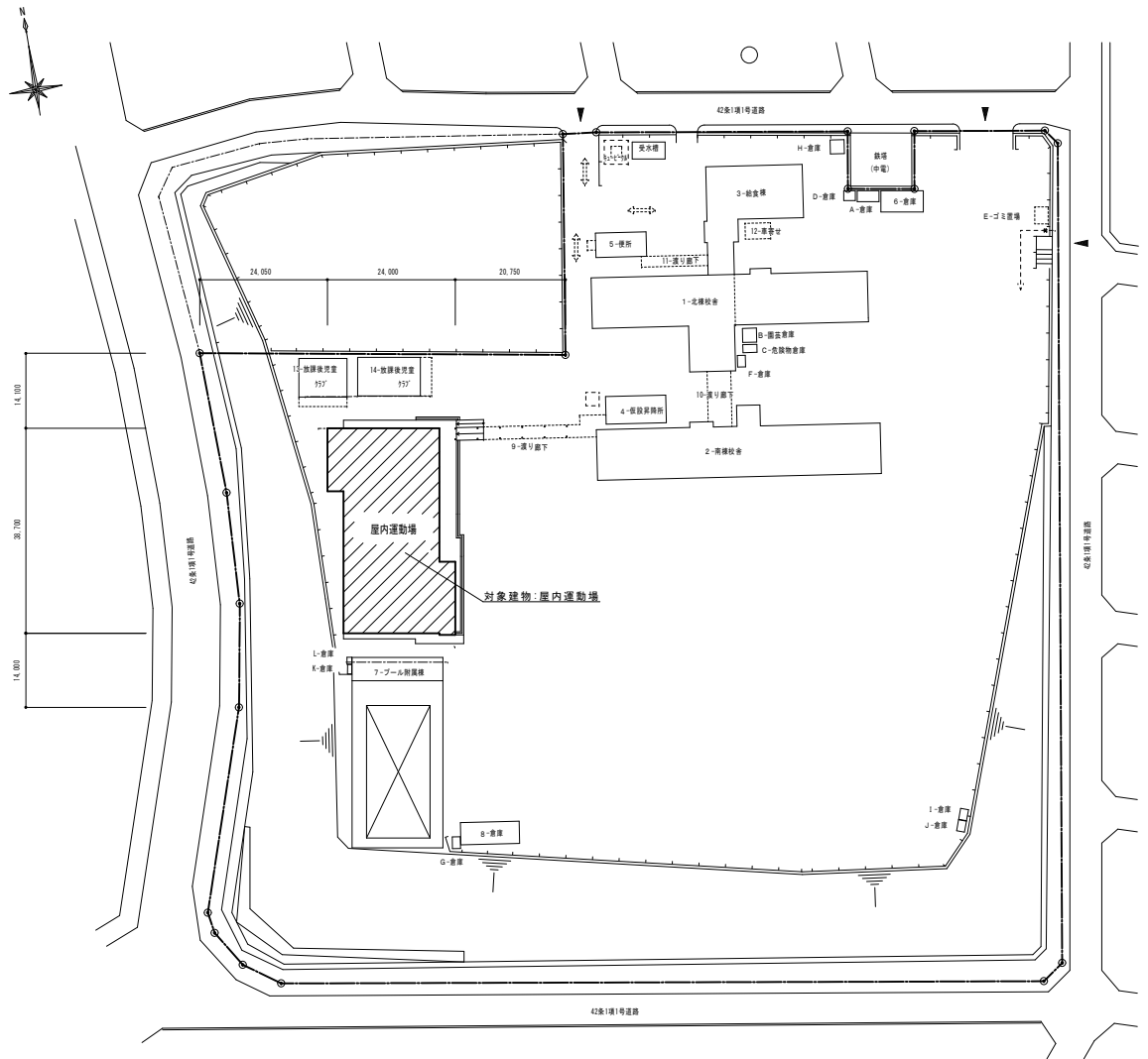
配置図 S=1/500
