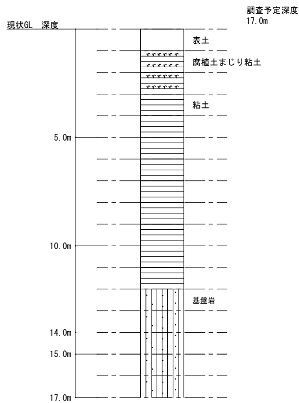
推定柱状図
