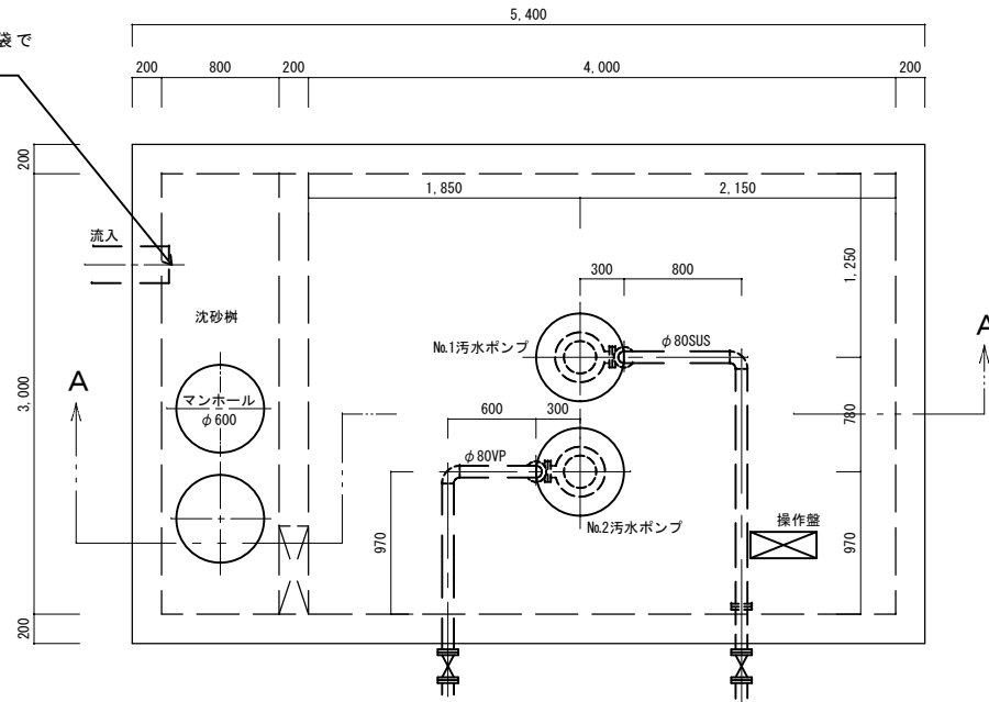
平面図
