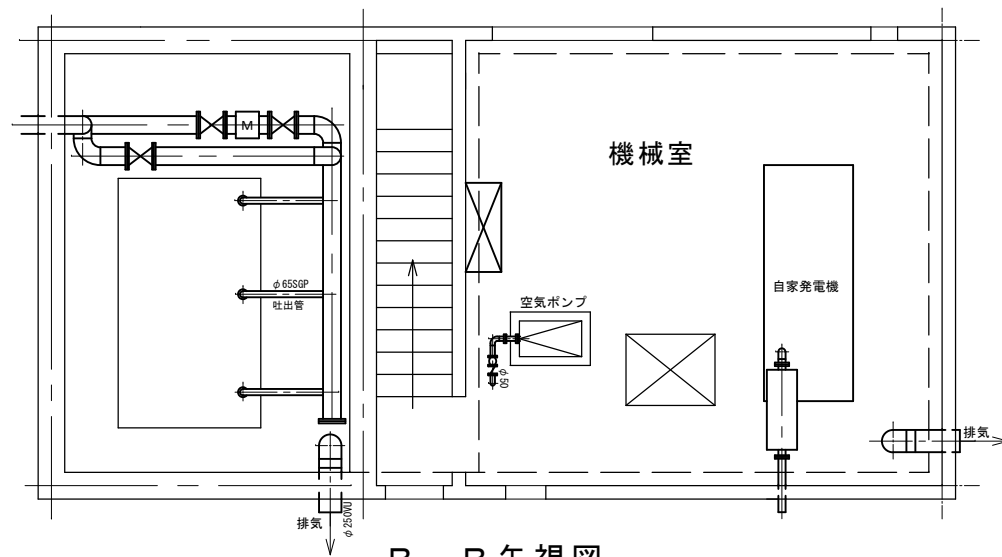
B - B 矢視図
