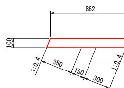
天端コンクリート S=1:20
