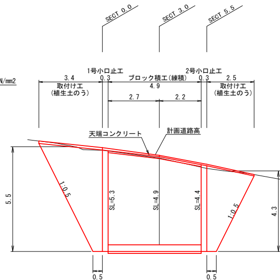
2号小口止工 SECT 5.5 S=1:50
