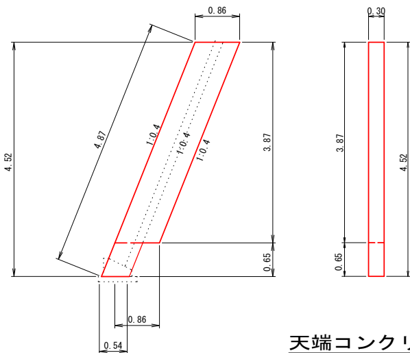
2号小口止工 SECT 5.5 S=1:50
