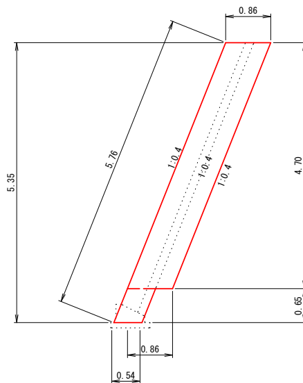
1号小口止工 SECT 0.0 S=1:50
