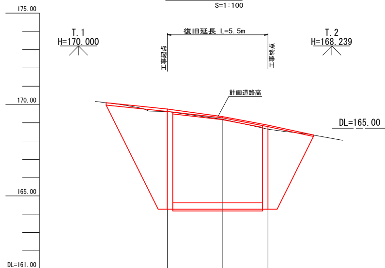
縦 断 図 S=1:100
