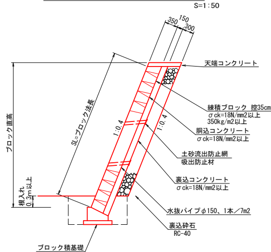
ブロック積工(練積) S=1:50
