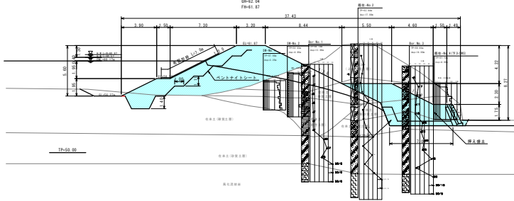
取水施設部断面図 S=1:200
