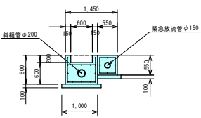
底樋 (PCa) 断面図 S=1:50
