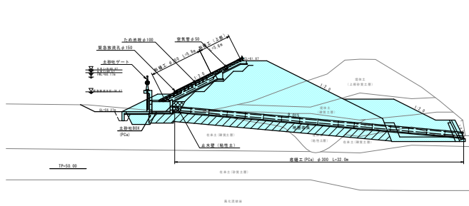
取水施設部断面図 S=1:200
