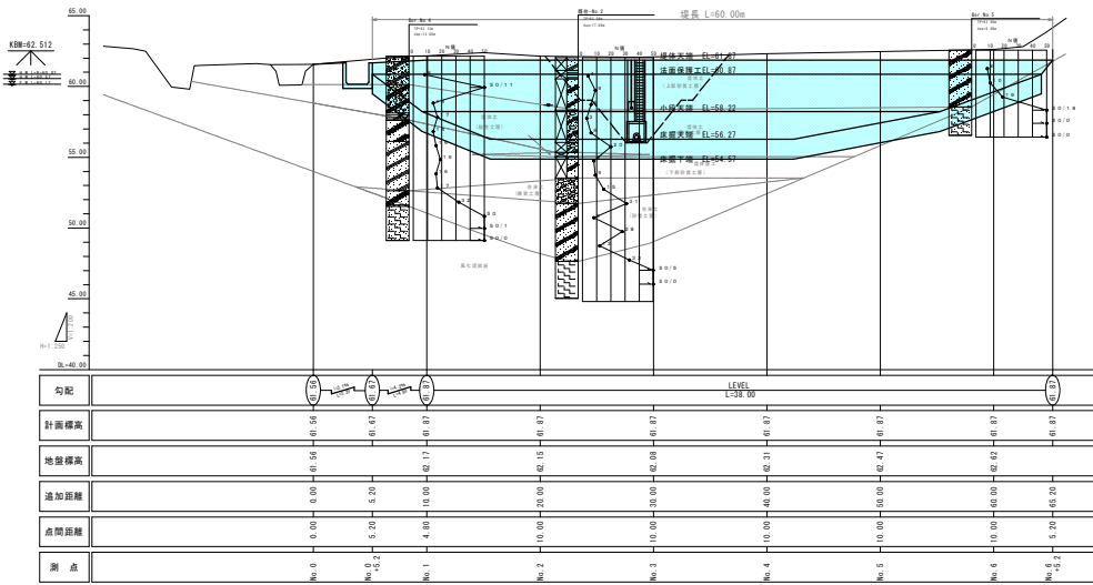
堤体縦断面図
