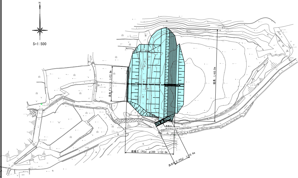
計画平面図 S=1:500
