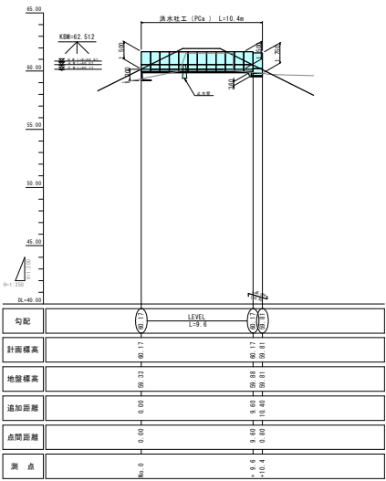
洪水吐縦断面図
