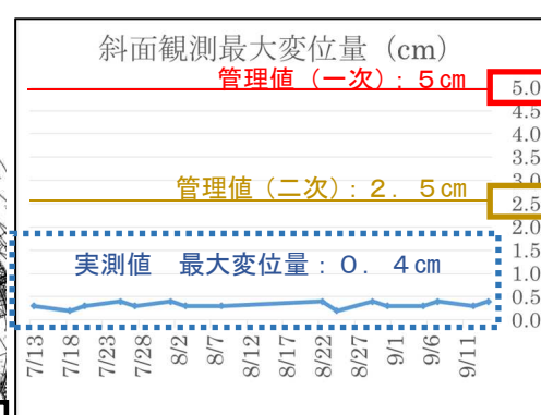
◆斜面変位の結果
