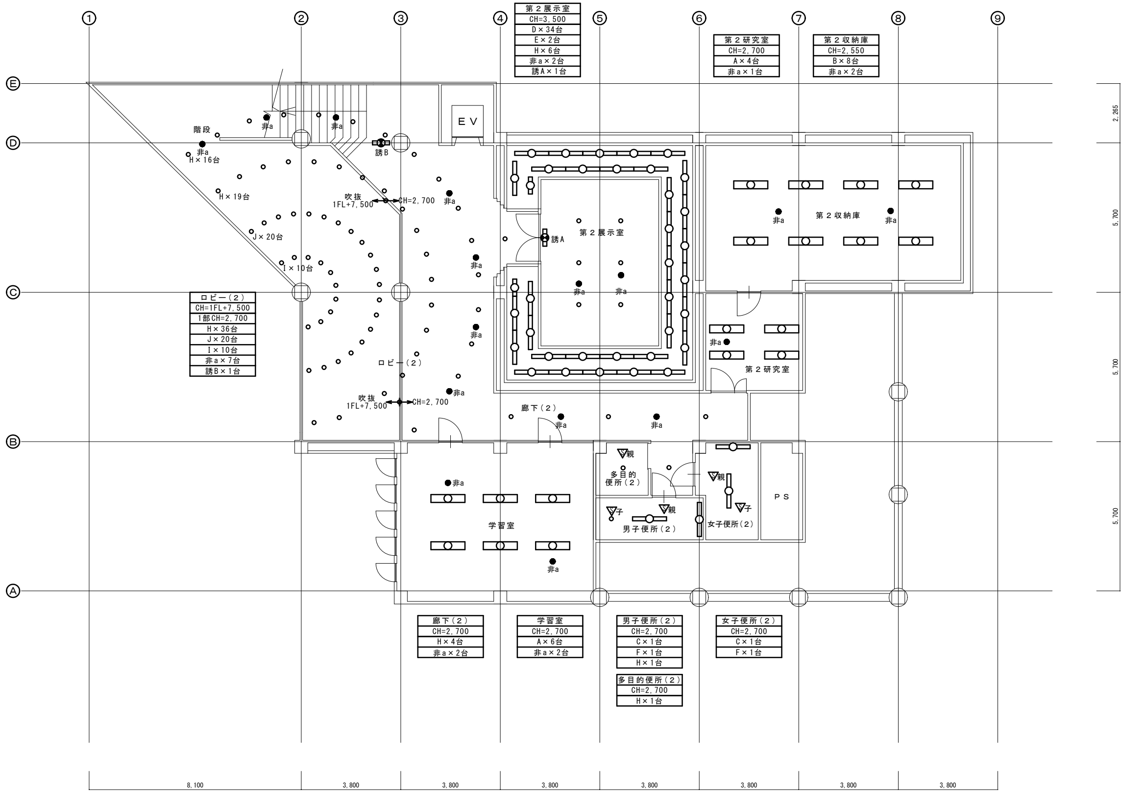
2 階平面図 1:100
