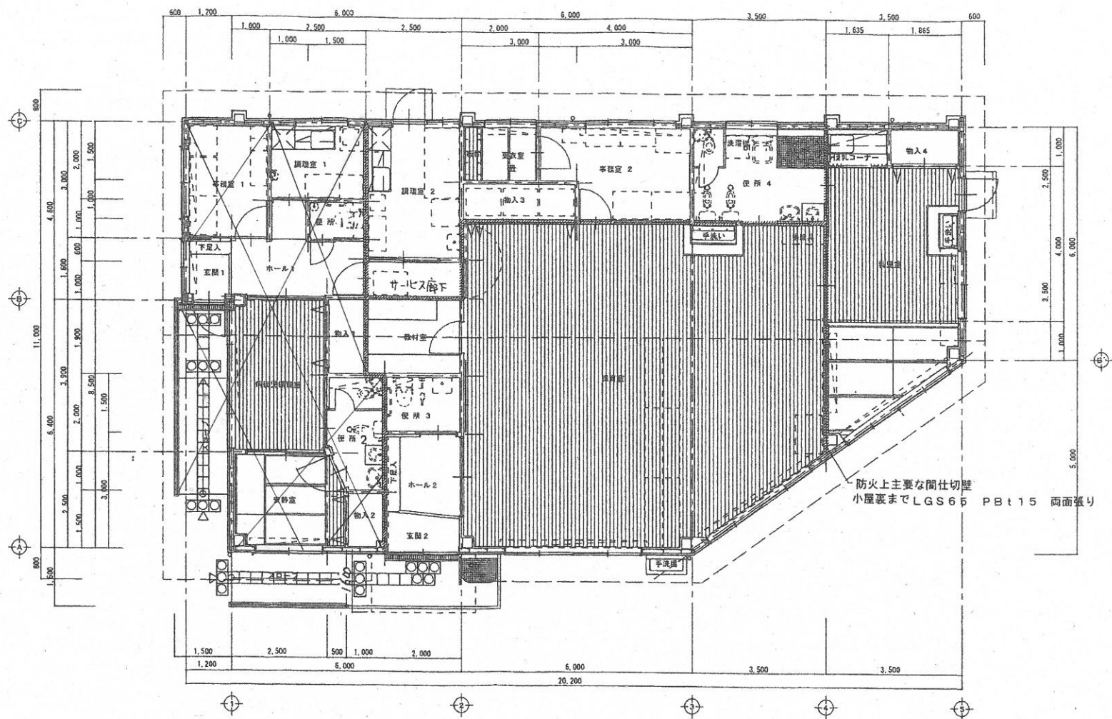
平面図図 S = 1 : 100
