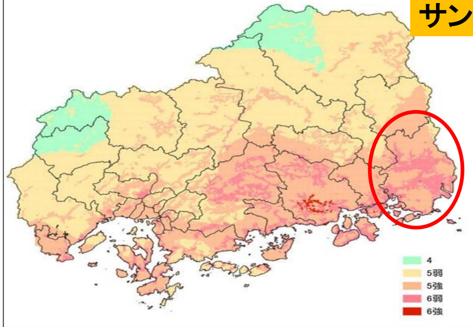
南海トラフ巨大地震(陸側ケース) 震度分布【令和7年県想定】
