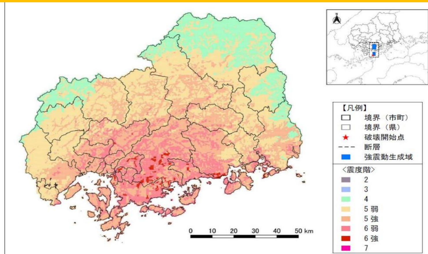
安芸灘～伊予灘～豊後水道(南から破壊開始) 震度分布
